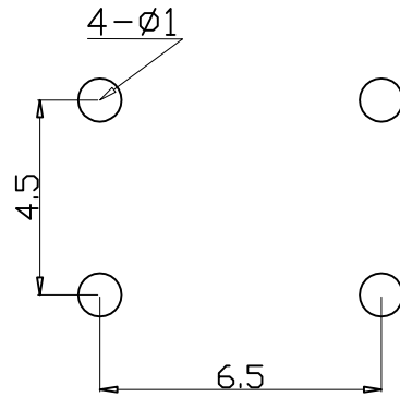
安装尺寸
