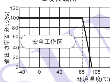
温度曲线图
