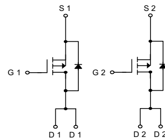
P-Channel MOSFET
