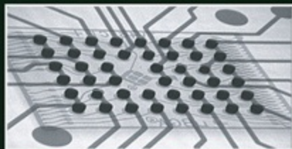
micro-BGA 焊点无空洞
