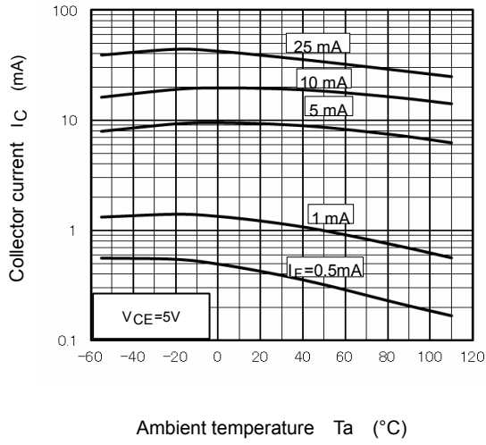
I_C - T_a
