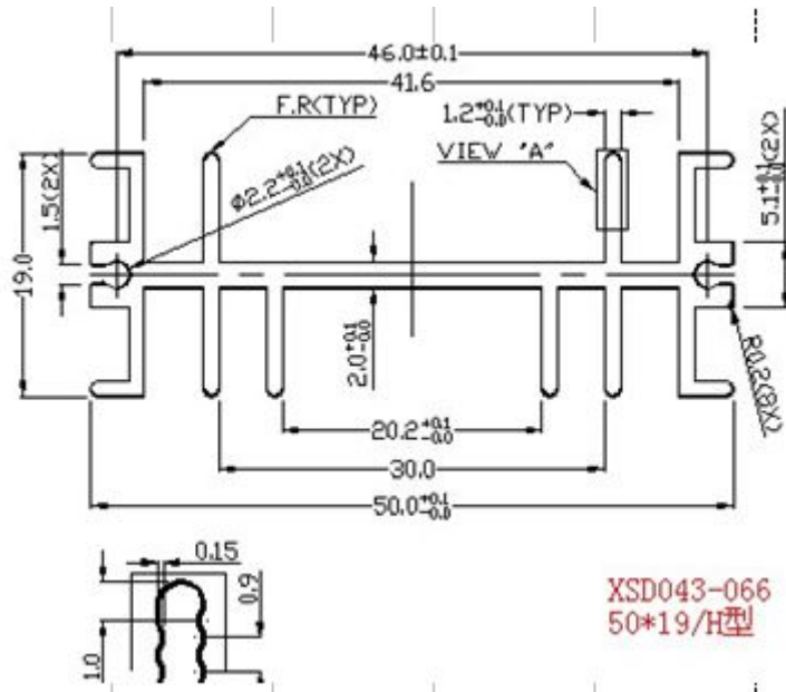
产品尺寸图
