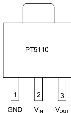
SOT89-3
