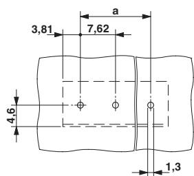
钻孔图
