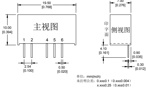
封装尺寸图
