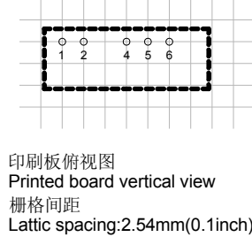
建议印刷板图
