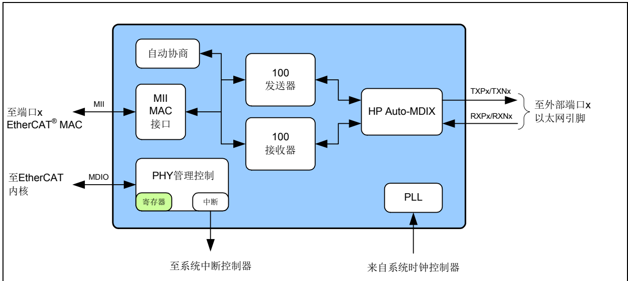
图 11-1: PHY 框图
