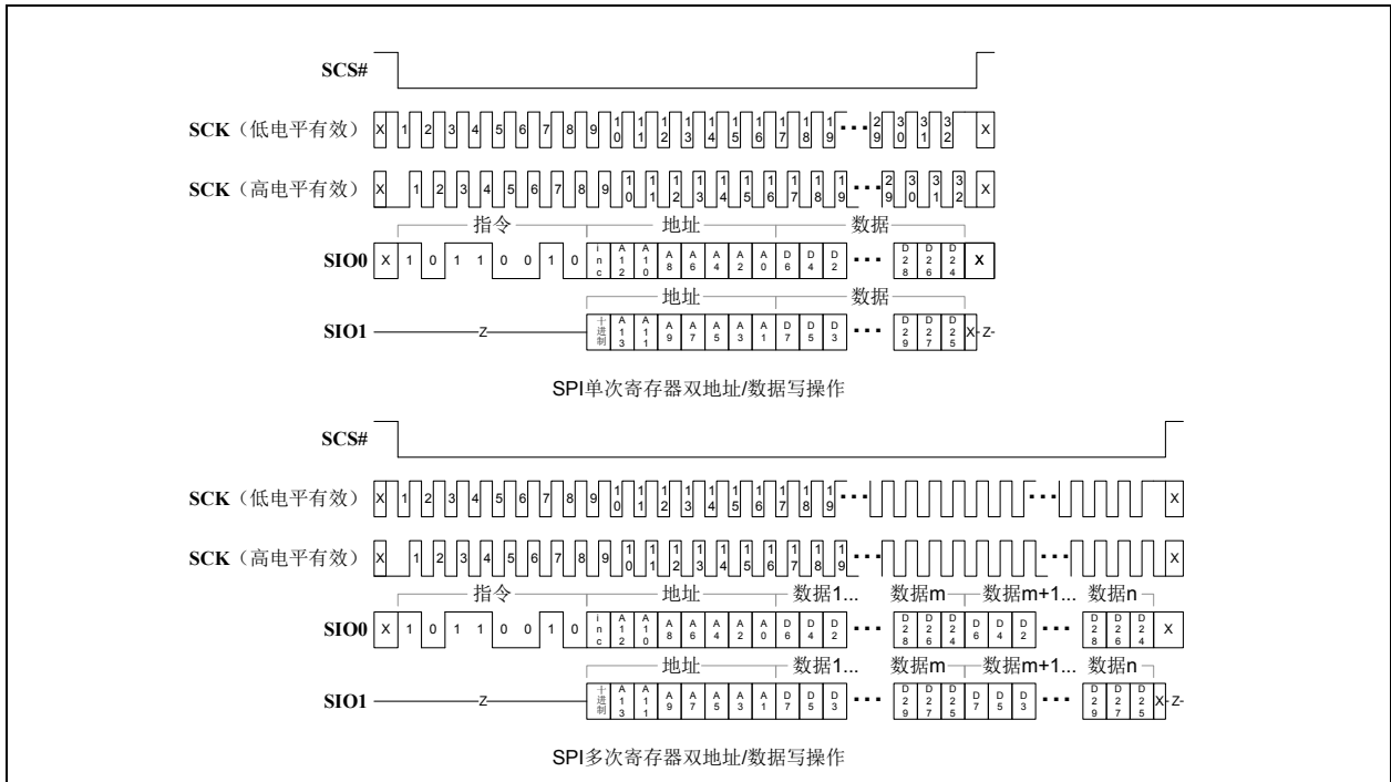
图 10-15: SPI双地址/数据写操作
