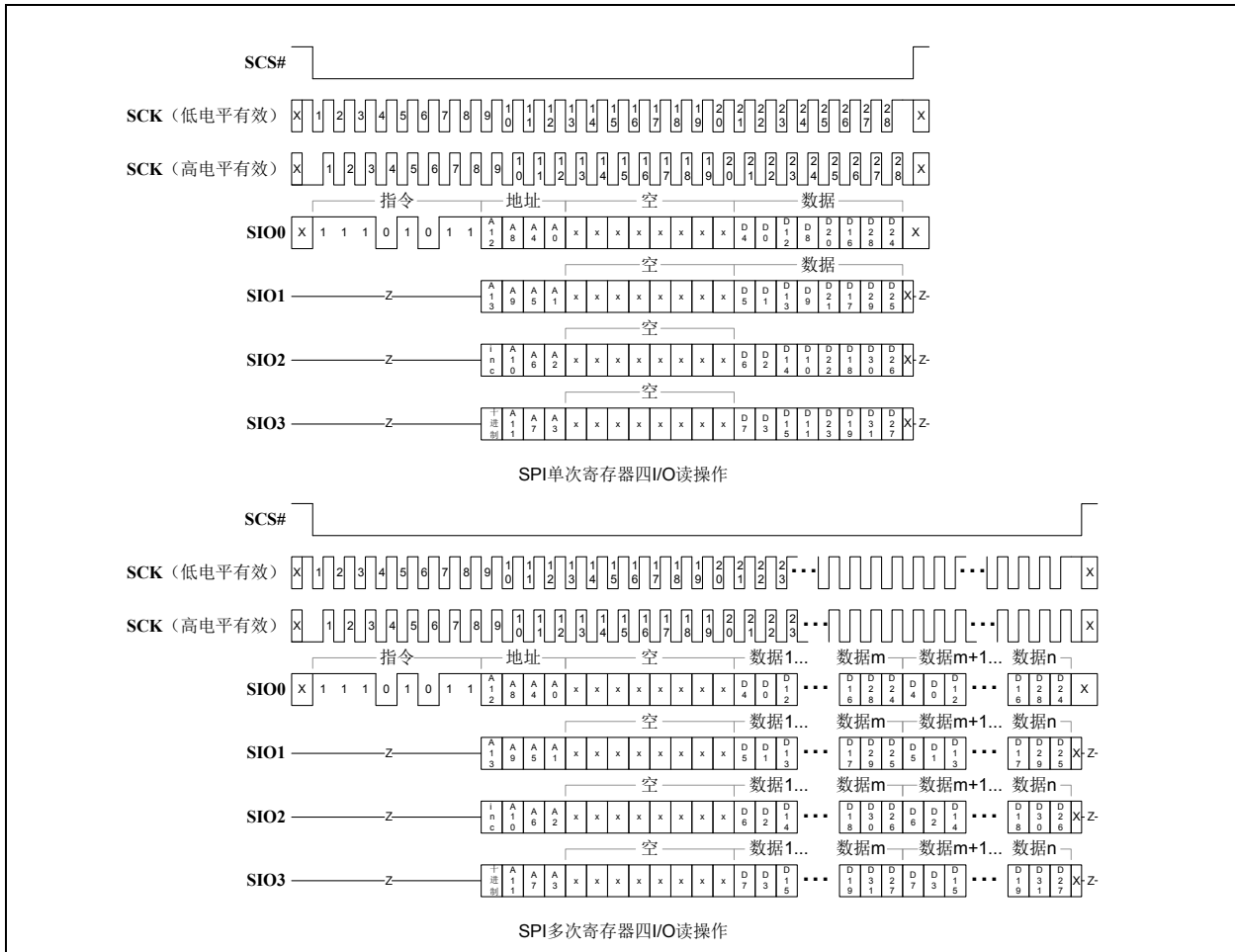
图 10-10: SPI 四 I/O 读操作
