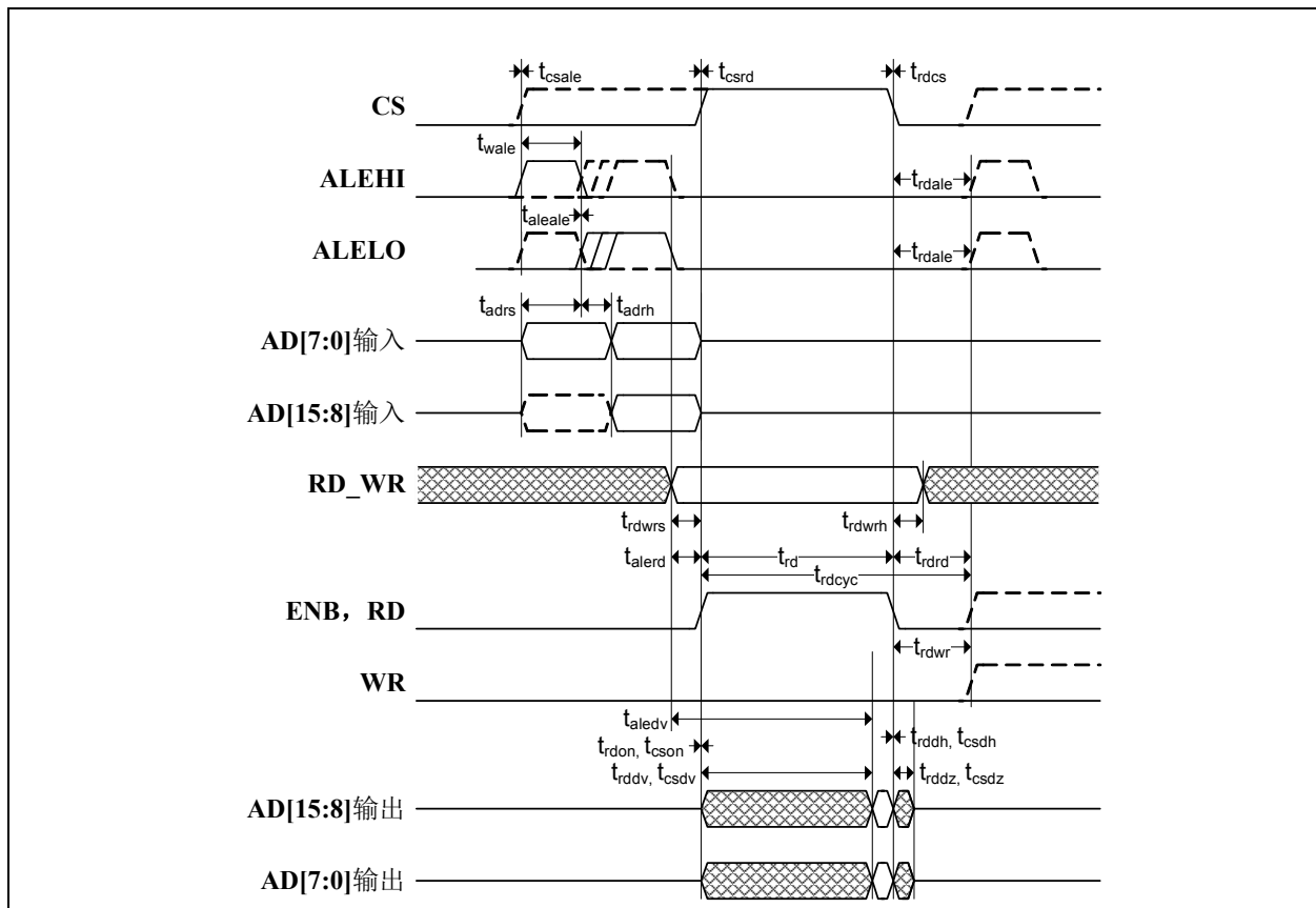
图9-21： 复用寻址读周期时序
