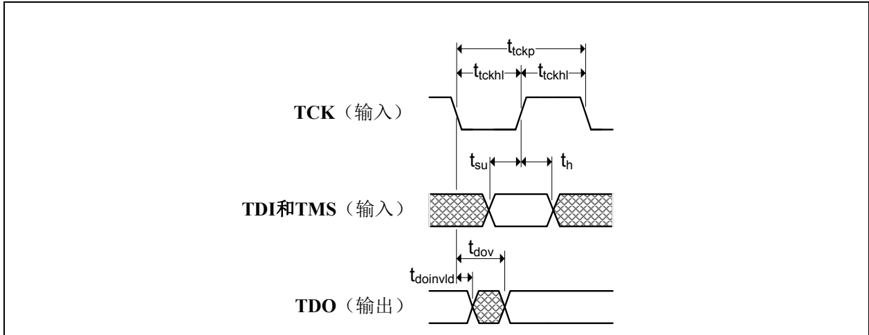
图17-1: JTAG时序
