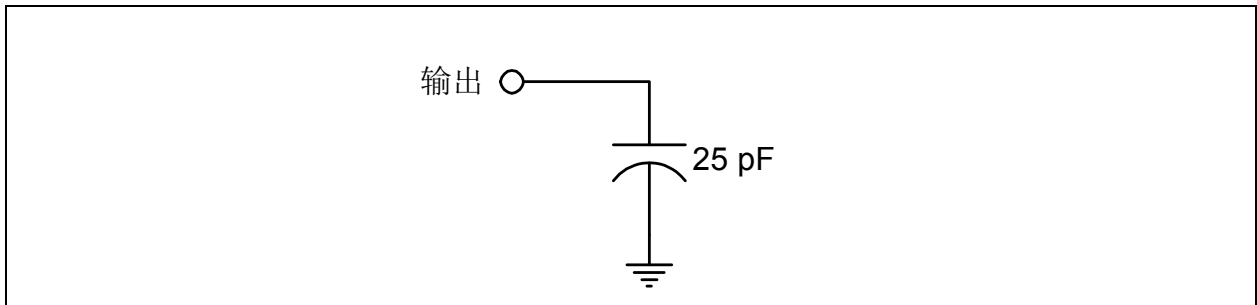
图18-1： 输出等效测试负载
