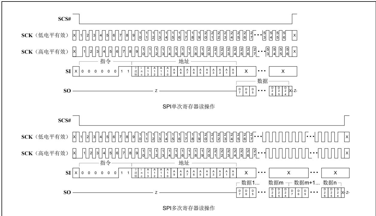
图10-4: SPI读操作
