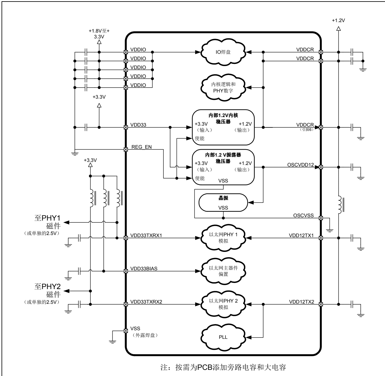
图4-2: 禁止稳压器时的电源连接
