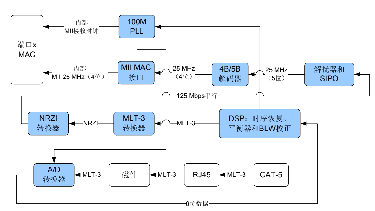
图11-3: 100BASE-TX接收数据路径
