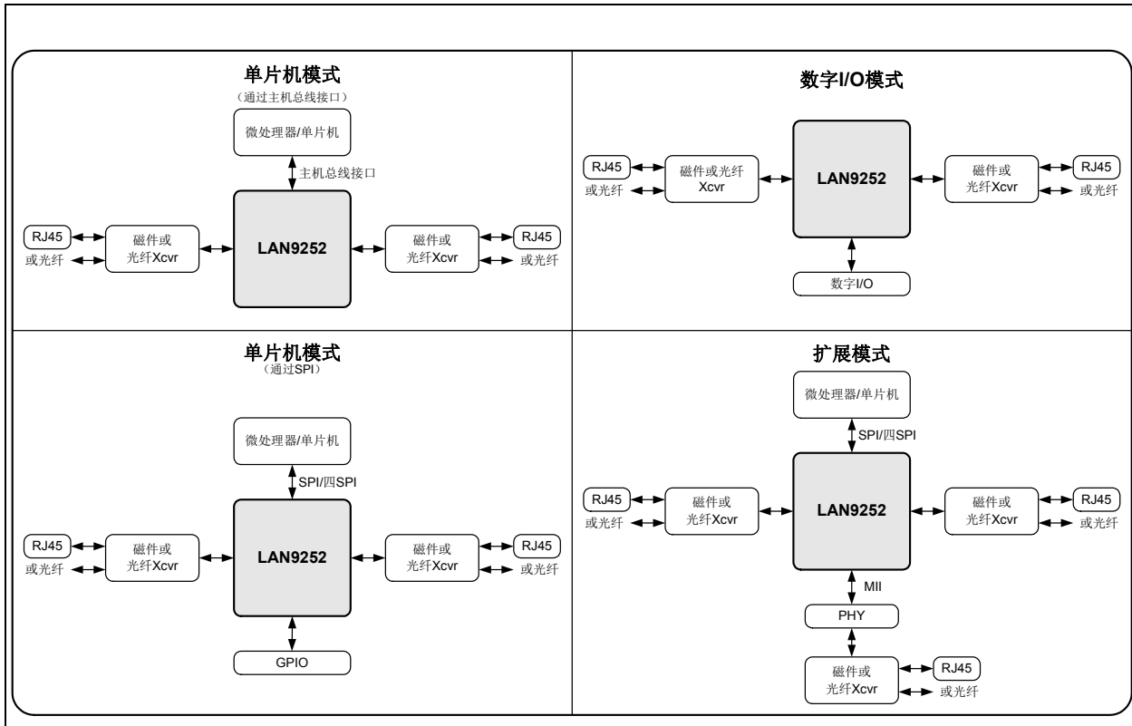
图2-3： 工作模式
