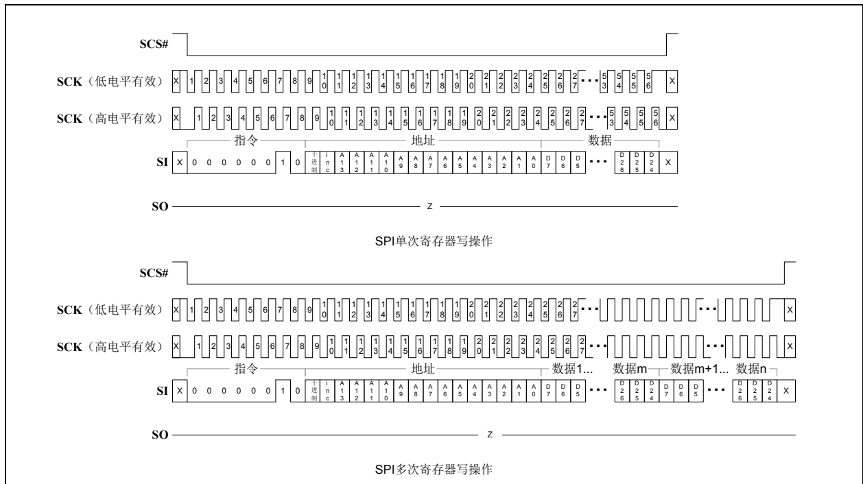
图10-11: SPI写
