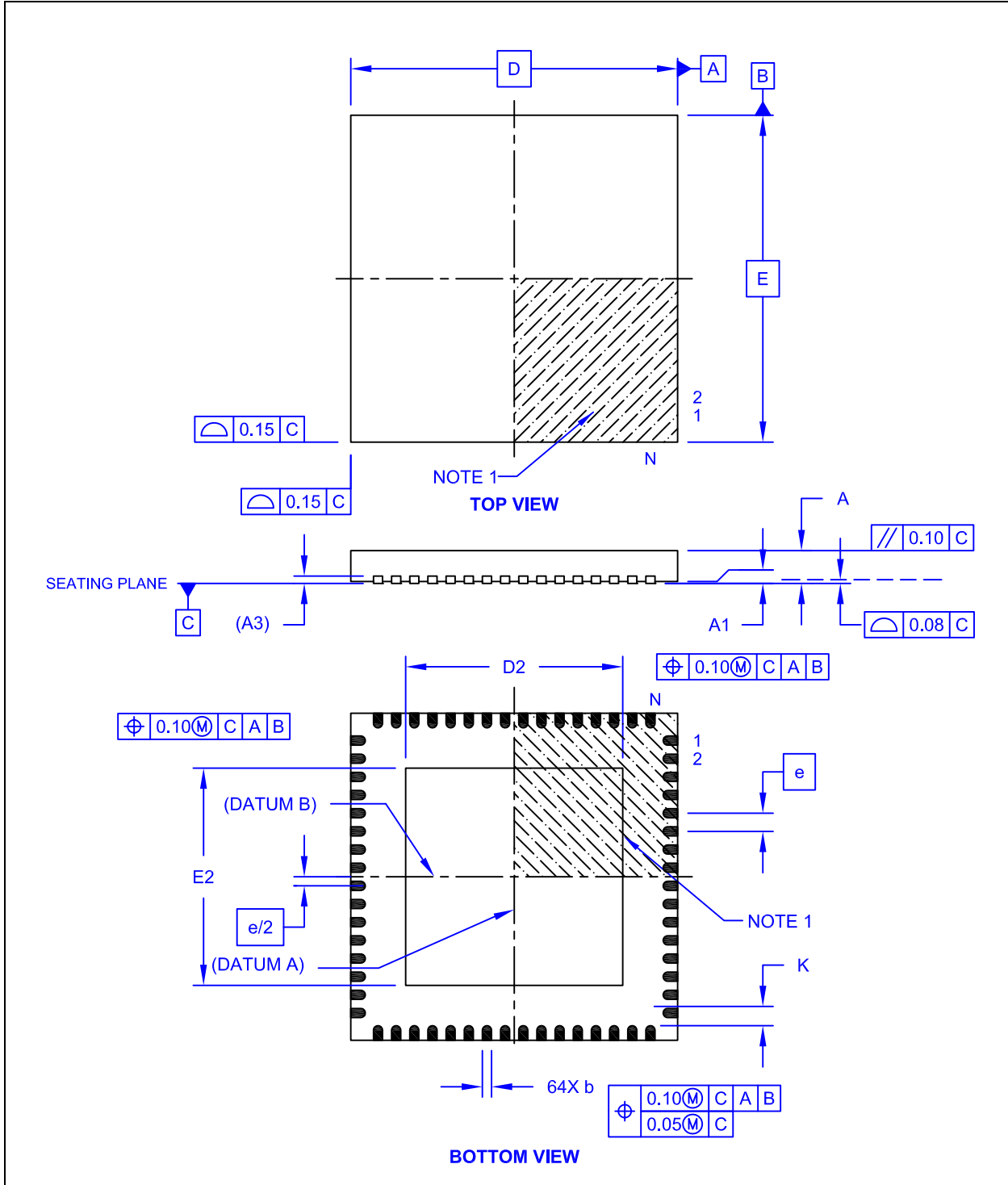
图 19-1: 64-QFN 封装
