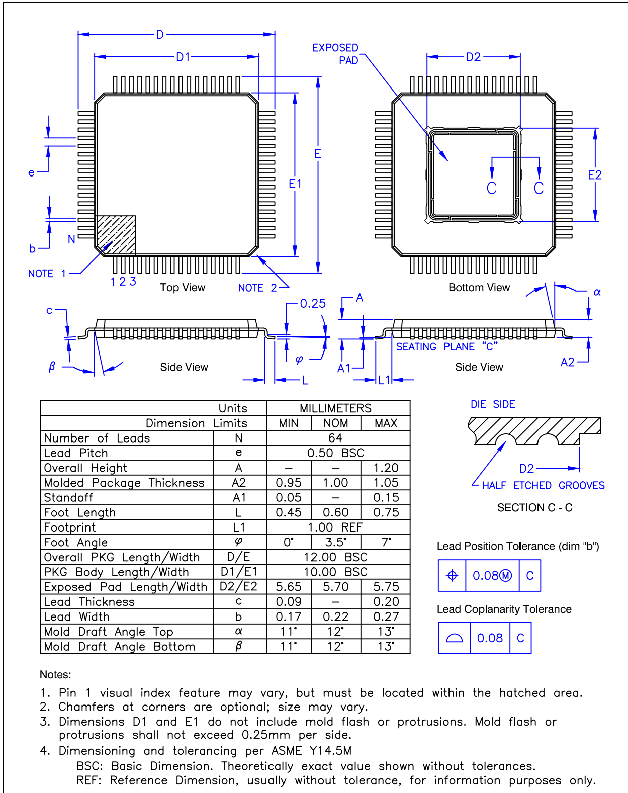
图19-3: 64-TQFP-EP封装
