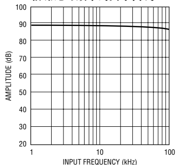
信噪比与频率的关系曲线
