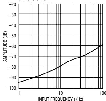
总谐波失真与输入频率的关系曲线
