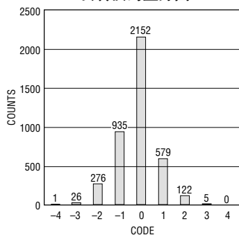
4096 次转换的直方图
