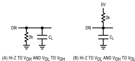
用于存取定时的负载电路
