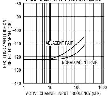
串扰与输入频率的关系曲线
