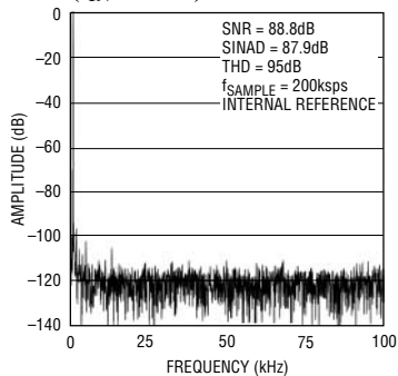
4096 点 FFT 曲线图 (f IN = 1kHz)
