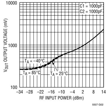
LTC5507 检波器典型特性， 100MHz， V_{CC} = 2.7V 至 6V
