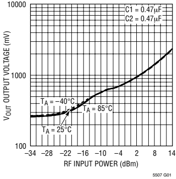
LTC5507 检波器典型特性， 100kHz， V_{CC} = 2.7V 至 6V
