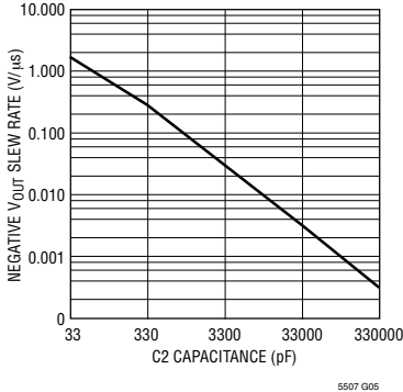
负 V_{OUT} 转换速率与 C2 电容 的关系曲线
