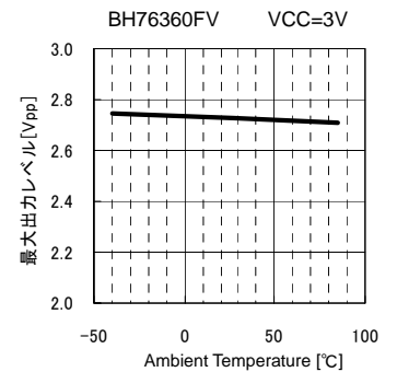
Fig.28 Vom vs. Ambient Temperature
