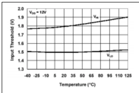
图 2-12: 输入阈值—温度关系曲线
