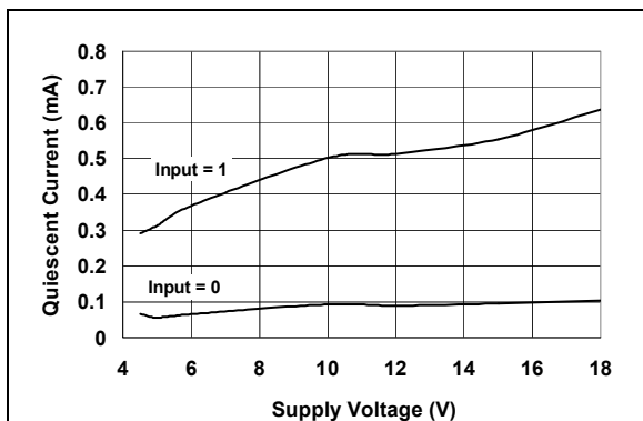
图 2-9: 静态电流—电源电压关系曲线
