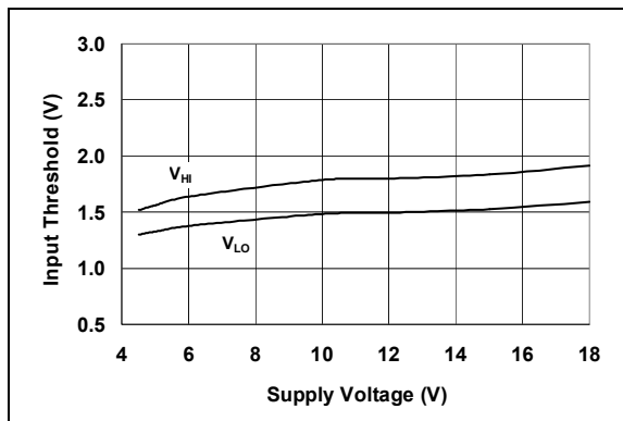
图 2-11: 输入阈值—电源电压关系曲线
