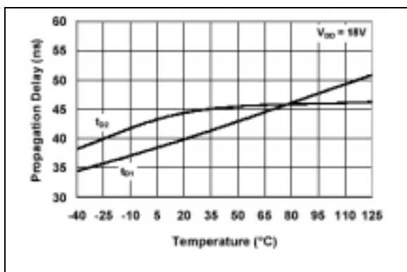
图 2-8: 传输延迟时间—温度关系曲线
