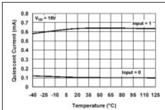
图 2-10: 静态电流—温度关系曲线
