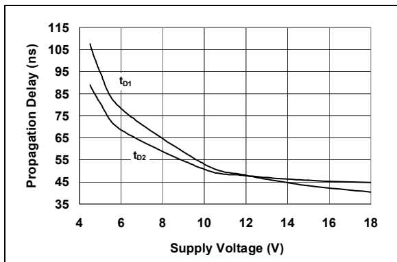
图 2-7: 传输延迟时间—电源电压关系曲线
