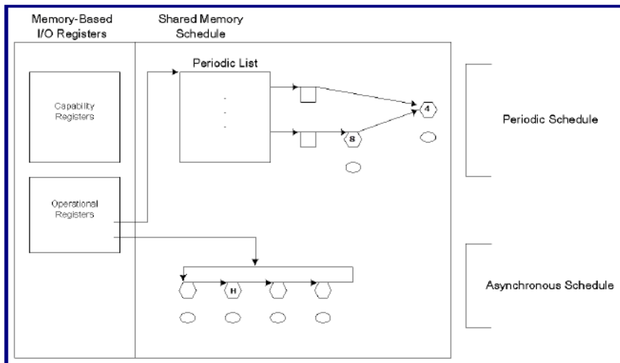
图 14-5 EHCI 数据传输调度表
