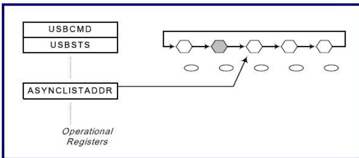
图14-7 异步调度表列表
