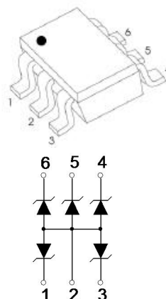
SOT-363
