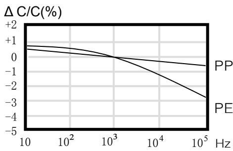
频率特性
