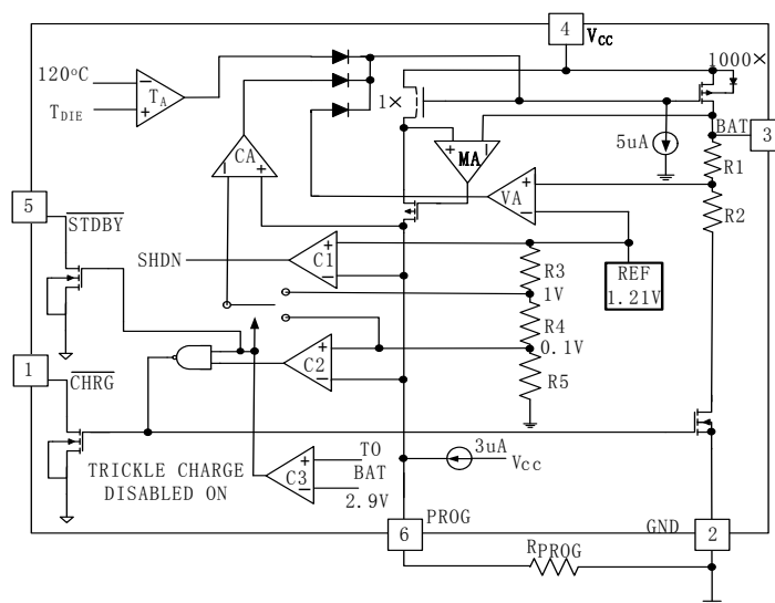
图 2 功能框图
