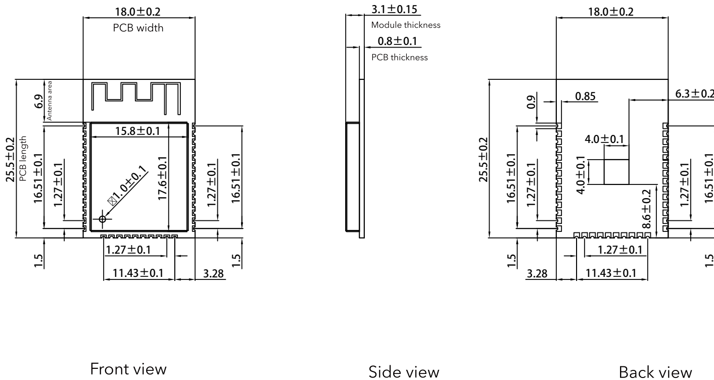
图 5: ESP-WROOM-32 尺寸
