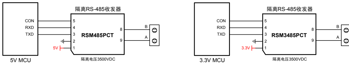
图 1 典型连接电路图
