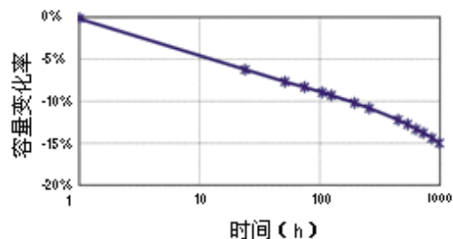
SP-Z 系列高温负荷特性
