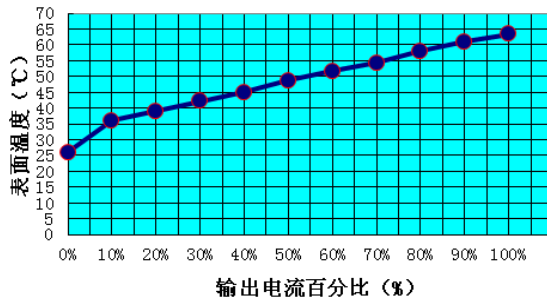
壳温VS输出负载曲线图
