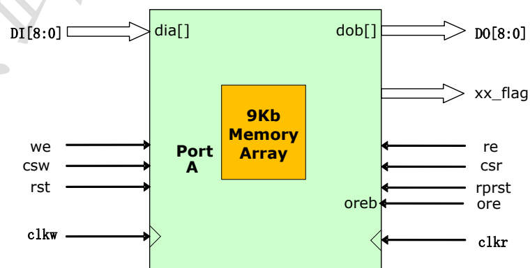
图 2-2-7 &lt;=9 位进/&lt;=9 位出 FIFO 模式
