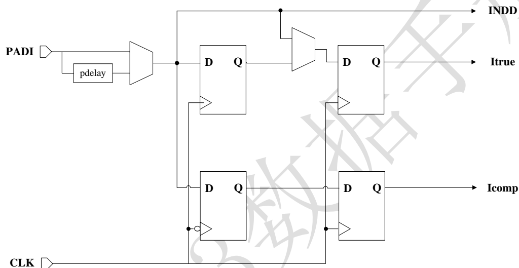
图 2-6-1: 输入寄存器框图
