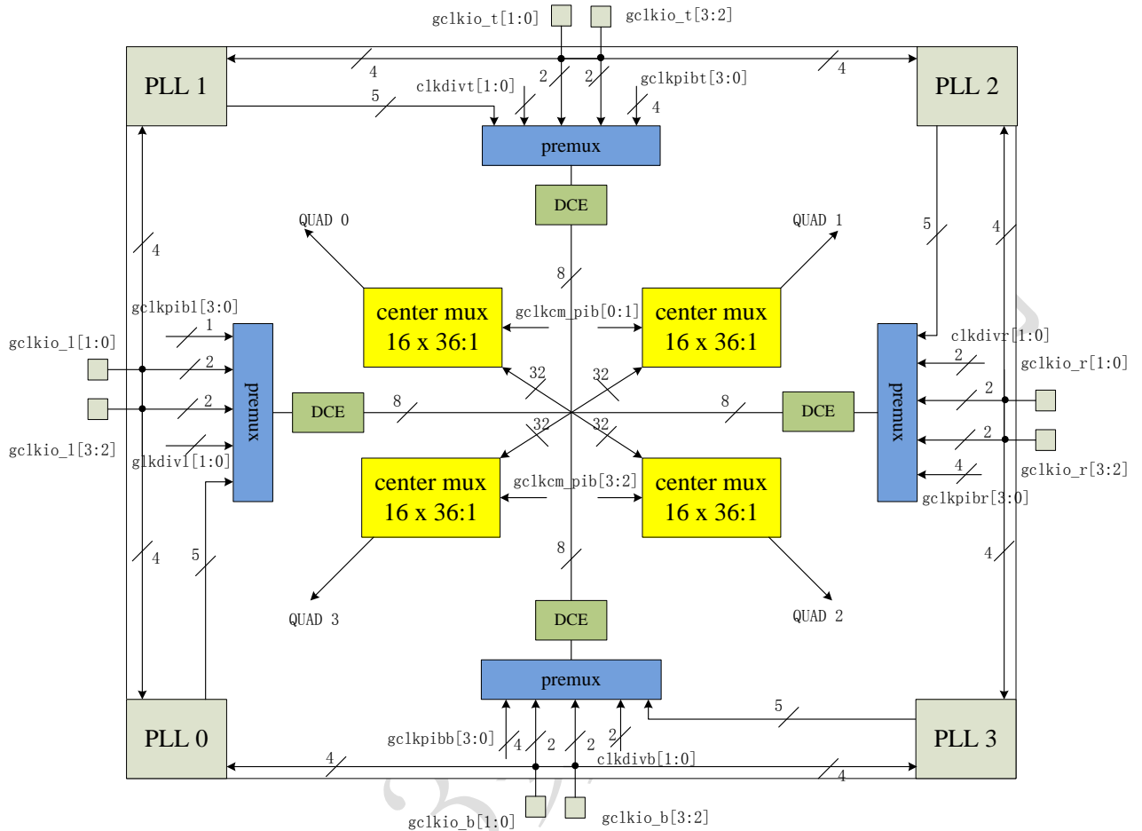
图 2-3-1: 全局时钟分布网络
