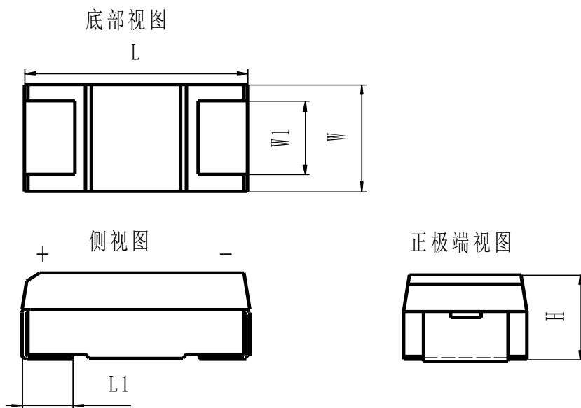
图 1 外形图
