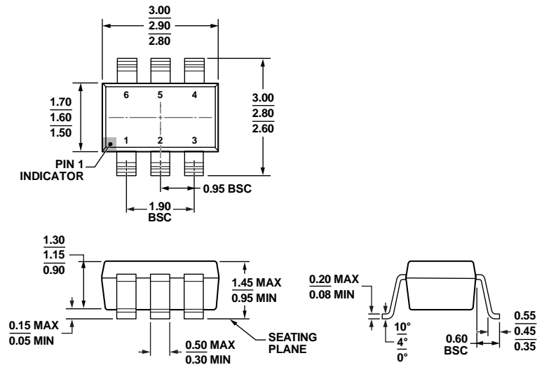
图45. 6引脚小型晶体管封装(SOT-23) (RJ-6) 图示尺寸单位: mm
