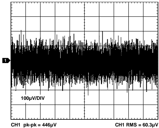
图22. ADR3450输出电压噪声(10 kHz至10 kHz)
