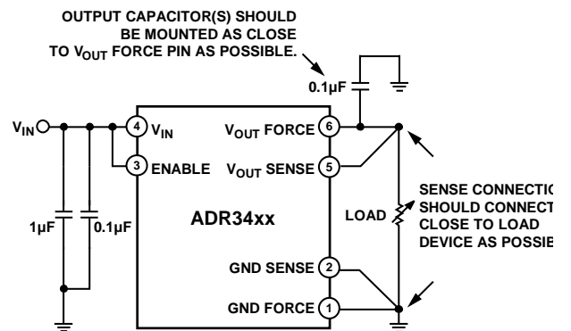
图41. 开尔文连接应用示例
