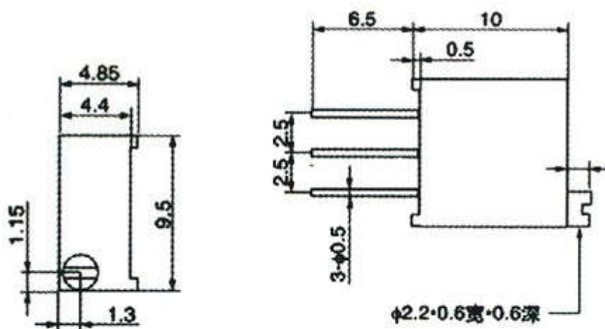
共有尺寸图
