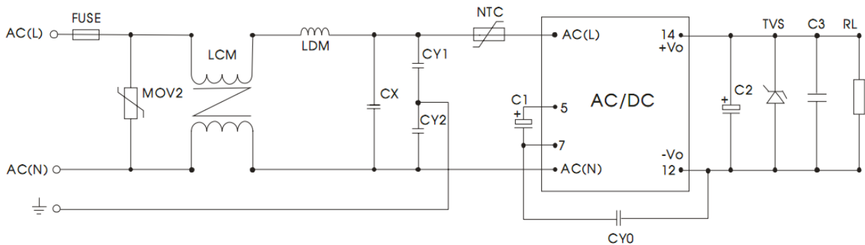
图 2: EMC 更高要求应用电路
