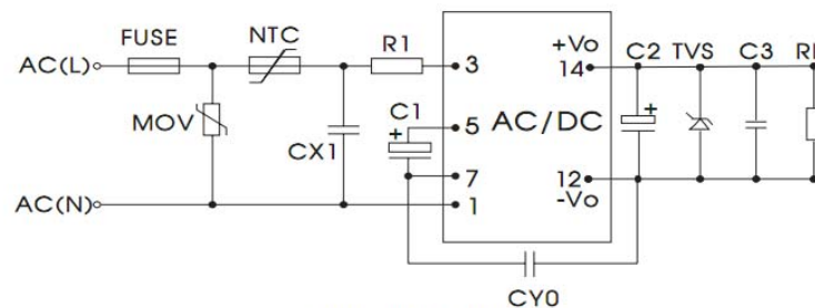
图 1：典型应用电路
