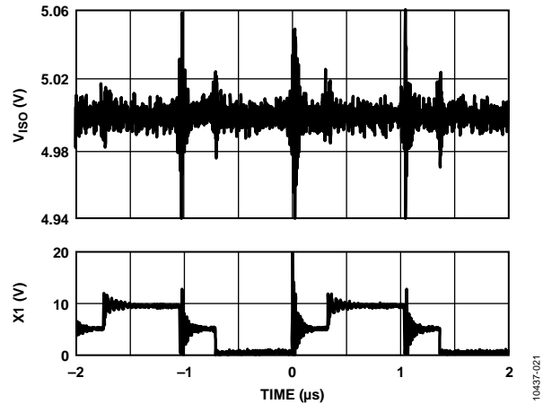
图27.典型 V_{ISO} 输出纹波(5V输入至5V输出, 开关频率 f_{SW} = 500 kHz, 负载为500 mA)
