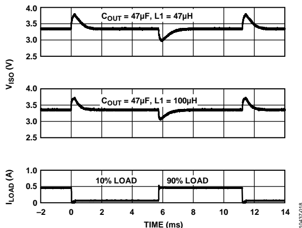
图21.典型 V_{ISO} 负载瞬态负载响应(5V输入至3.3 V输出, 开关频率 f_{SW} = 500 kHz, 负载为500 mA的10%至90%负载)
