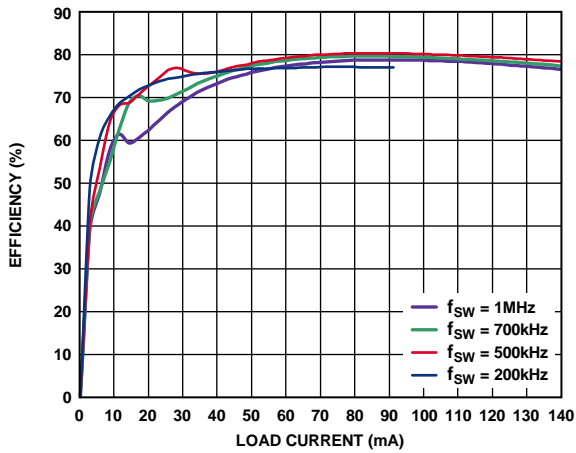
图11. 5 V输入至15 V输出时, 不同开关频率下的效率 (1:3 Coilcraft变压器(JA4650-BL))
