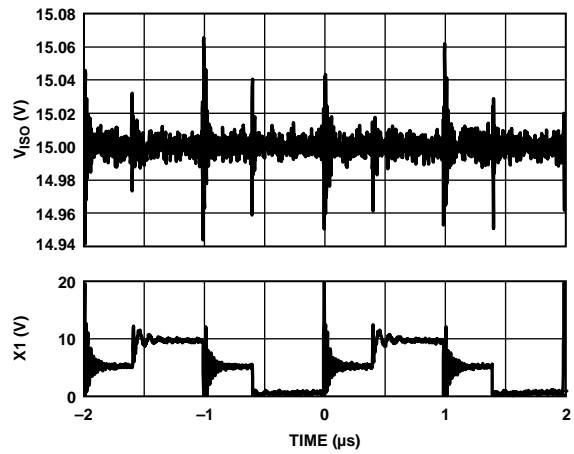
图30.典型 V_{ISO} 输出纹波(5V输入至15 V输出, 开关频率 f_{SW} = 500 kHz, 负载为100 mA)
