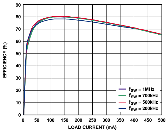
图6. 5 V输入至5 V输出时，不同开关频率下的典型效率(1:2 Halo变压器(TGSAD-260V6LF))
