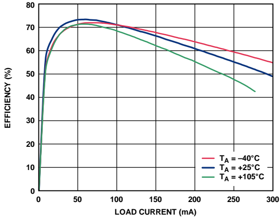
图10. 开关频率 f_{sw}=500 kHz时, 在整个温度范围内的效率 (3.3 V输入至5 V输出, 1:3 Halo变压器(TGSAD-290V6LF))
