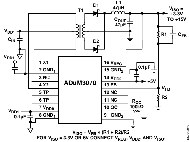
图31.单电源
