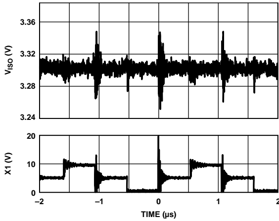
图28.典型 V_{ISO} 输出纹波(5V输入至3.3 V输出, 开关频率 f_{SW} = 500 kHz, 负载为500 mA)
