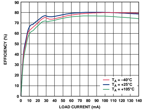
图13. 开关频率 f_{sw}=500 kHz时, 在整个温度范围内的效率 (5 V输入至15 V输出, 1:3 Coilcraft变压器(JA4650-BL))
