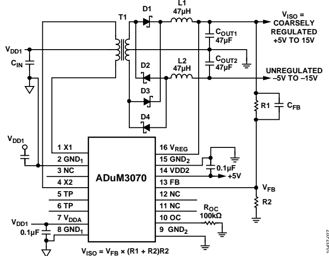
图33.正电源及无调节负电源
