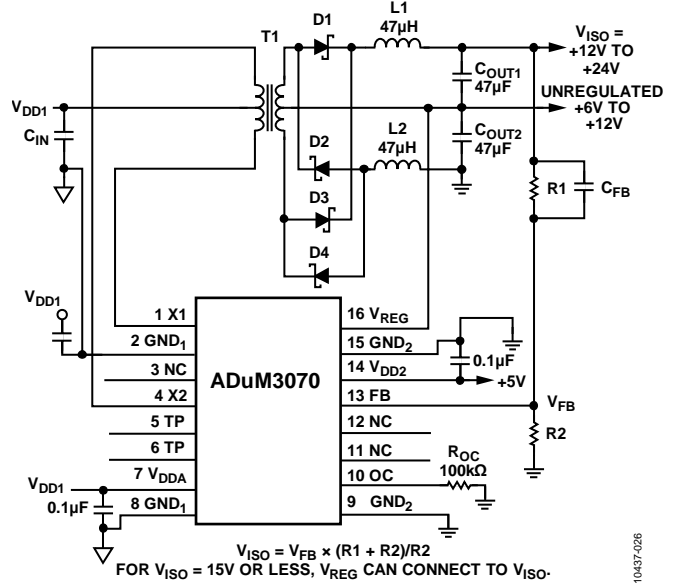
图32.双电源
