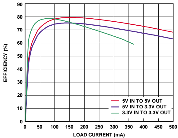
图8. 开关频率 f_{sw}=500\text{ kHz} 时，单电源供电效率(1:2 Coilcraft变压器(JA4631-BL))
