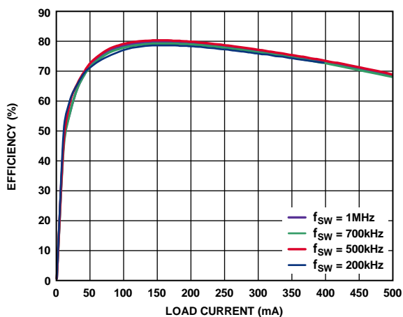
图5. 5 V输入至5 V输出时，不同开关频率下的典型效率(1:2 Coilcraft变压器(JA4631-BL))
