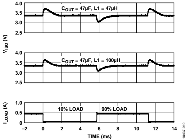
图23.典型 V_{ISO} 负载瞬态响应(3.3V输入至3.3V输出, 开关频率 f_{SW} = 500 kHz, 负载为250 mA的10%至90%)
