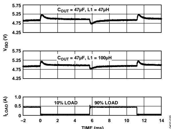
图20.典型 V_{ISO} 负载瞬态响应(5V输入至5 V输出, 开关频率 f_{SW} = 500 kHz, 负载为500 mA的10%至90%, 0.1 µF反馈电容)
