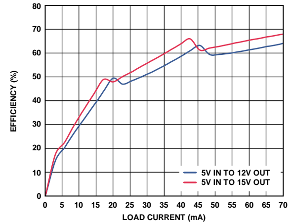
图14. 开关频率 f_{sw}=500 kHz时, 双电源供电效率 (1:5 Coilcraft变压器(KA4976-AL))
