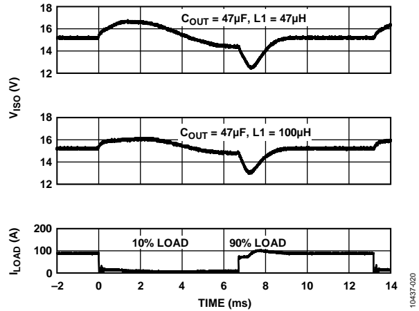
图25.典型 V_{ISO} 负载瞬态响应(5V输入至15V输出, 开关频率 f_{SW} = 500 kHz, 负载为100 mA的10%至90%)
