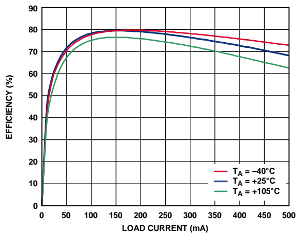
图7. 开关频率 f_{sw}=500\text{ kHz} 时，在整个温度范围内的效率(5 V输入至5 V输出，1:2 Coilcraft变压器(JA4631-BL))
