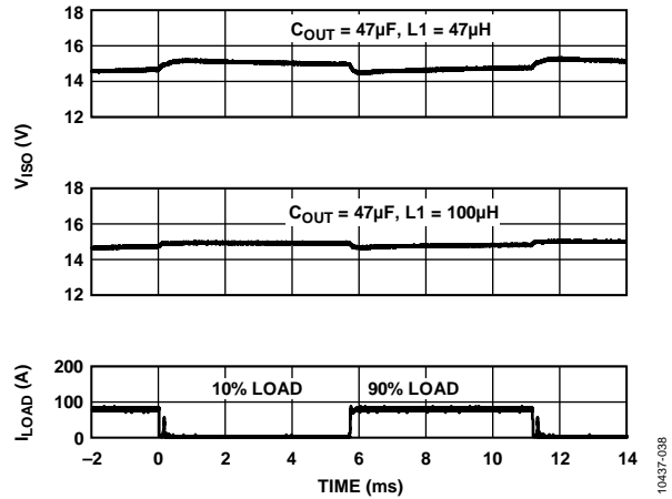
图26.典型 V_{ISO} 负载瞬态响应(5V输入至15V输出, 开关频率 f_{SW} = 500 kHz, 负载为100 mA的10%至90%, 0.1 \mu F反馈电容)
