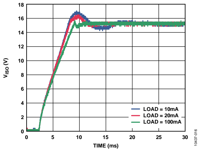
图18.典型 V_{ISO} 启动(5 V输入至15 V输出, 10 mA、20 mA和100 mA输出负载)
