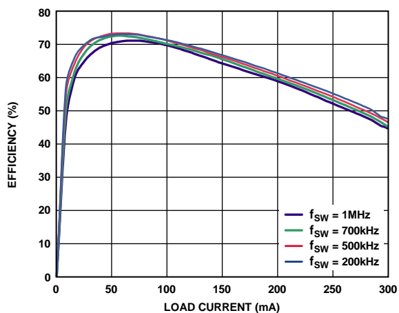
图9. 3.3 V输入至5 V输出时，不同开关频率下的典型效率(1:3 Halo变压器(TGSAD-290V6LF))
