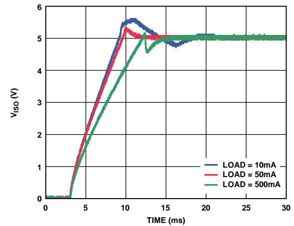
图15. 典型 V_{iso} 启动(5 V输入至5 V输出, 10 mA、50 mA和500 mA输出负载)
