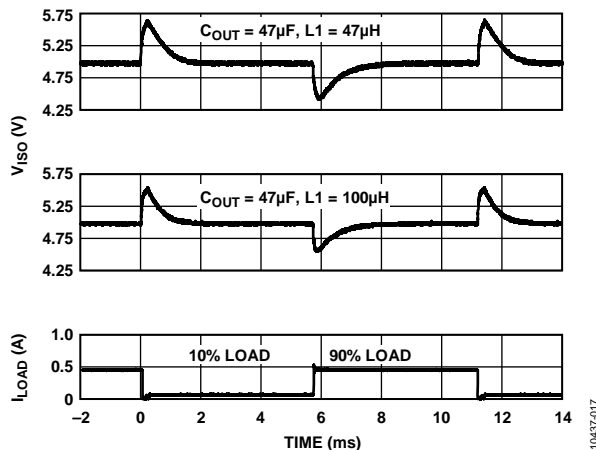
图19.典型 V_{ISO} 负载瞬态响应(5V输入至5 V输出, 开关频率 f_{SW} = 500 kHz, 负载为500 mA的10%至90%)
