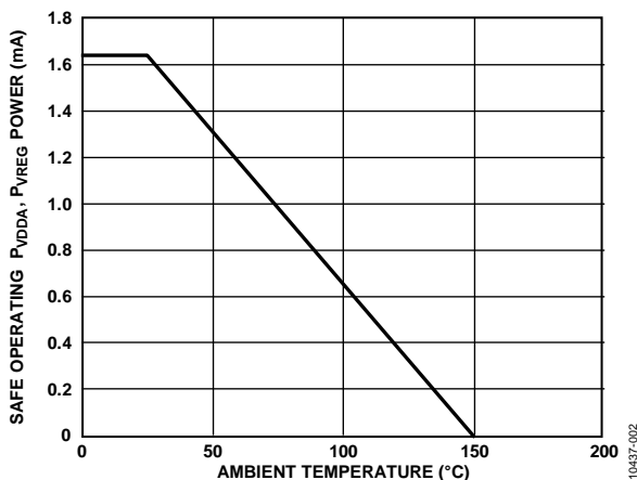
图2.热减额曲线，依据DIN V VDE V 0884-10获得的安全限值与环境温度的关系
