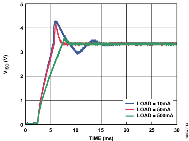
图16.典型 V_{ISO} 启动(5 V输入至3.3 V输出, 10 mA、50 mA和500 mA输出负载)
