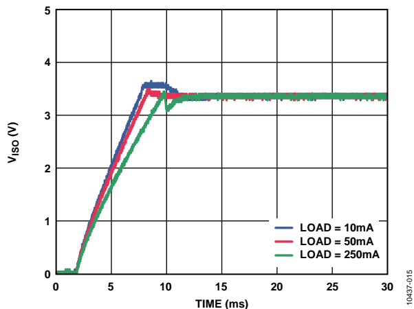
图17.典型 V_{ISO} 启动(3.3 V输入至3.3 V输出, 10 mA、50 mA和250 mA输出负载)
