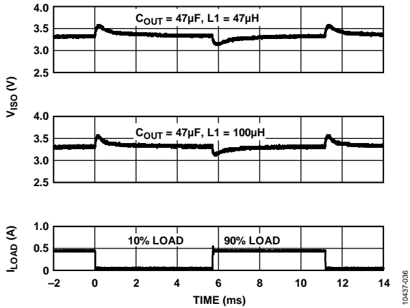
图22.典型 V_{ISO} 负载瞬态响应(5V输入至3.3V输出, 开关频率 f_{SW} = 500 kHz, 负载为500 mA的10%至90%负载, 0.1 \mu F反馈电容)
