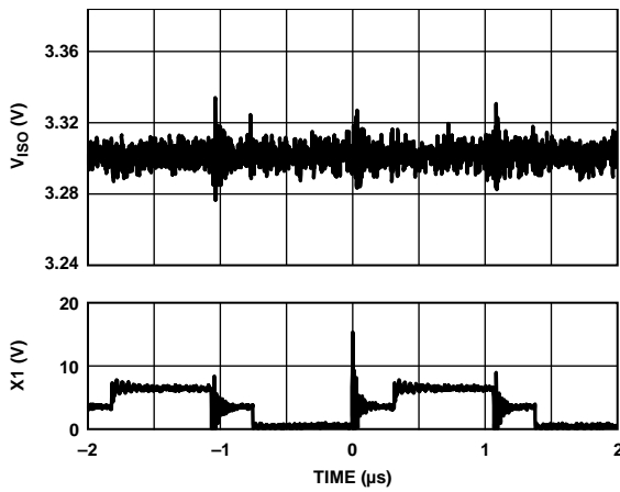
图29.典型 V_{ISO} 输出纹波(3.3 V输入至3.3 V输出, 开关频率 f_{SW} = 500 kHz, 负载为250 mA)
