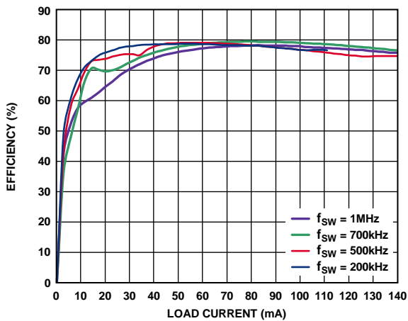
图12. 5 V输入至15 V输出时, 不同开关频率下的效率 (1:3 Halo变压器(TGSAD-290V6LF))
