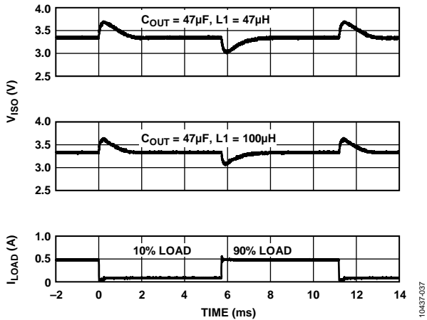
图24.典型 V_{ISO} 负载瞬态响应(3.3V输入至3.3V输出, 开关频率 f_{SW} = 500 kHz, 负载为250 mA的10%至90%, 0.1 \mu F反馈电容)
