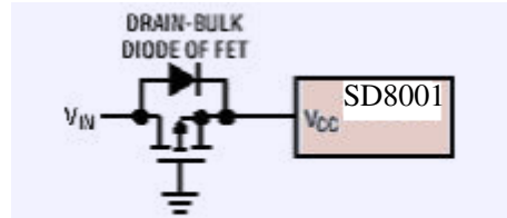
图 6: 低损耗输入反向极性保护
