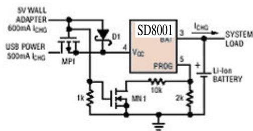
图 7: 交流适配器与USB电源组合
