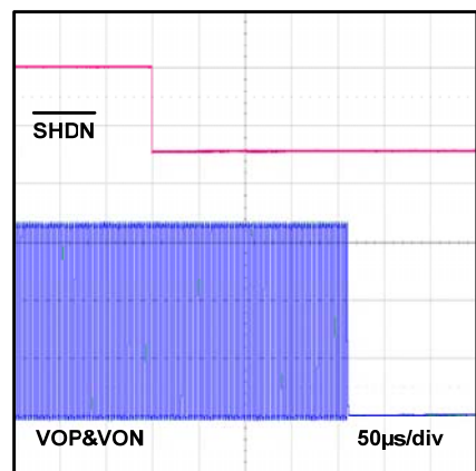
关断时序
