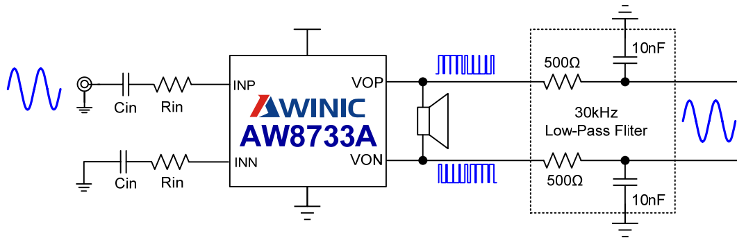
图 4 AW8733A 测试电路图
