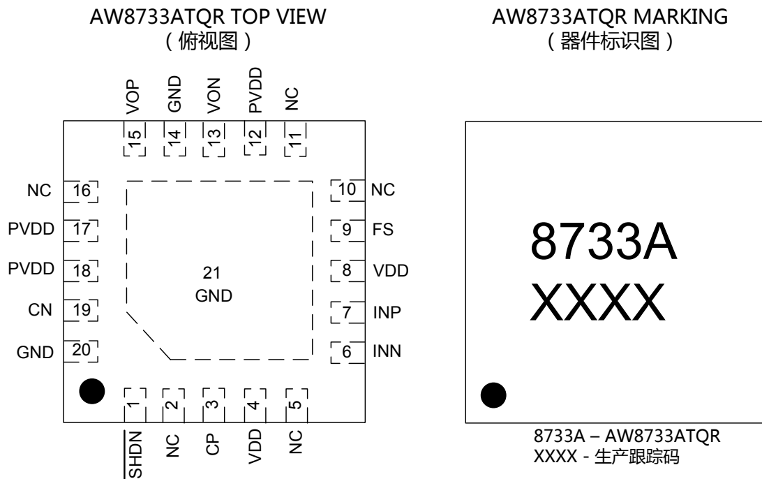
图 1 AW8733ATQR 引脚分布俯视图及器件标识图
