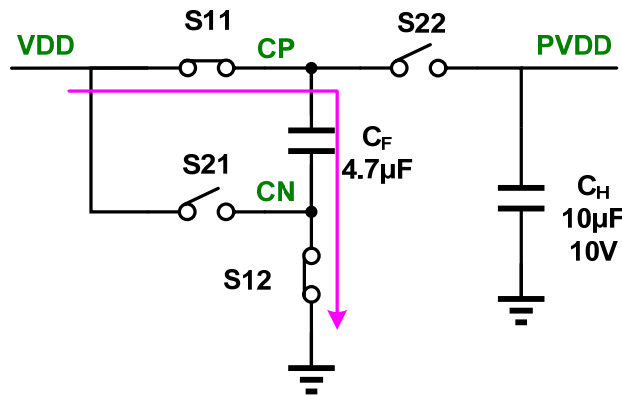
图 13 Φ1: Flying 电容充电
