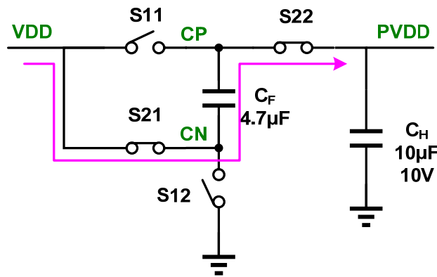
图 14 Φ2: Flying 电容电荷转移到输出电容 C_H
