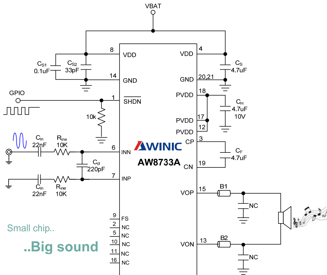
图2 AW8733A 单端输入方式典型应用图（注1）
