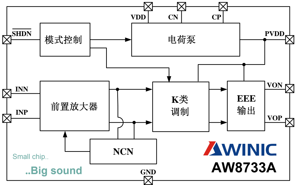
图 6 AW8733A 功能框图
