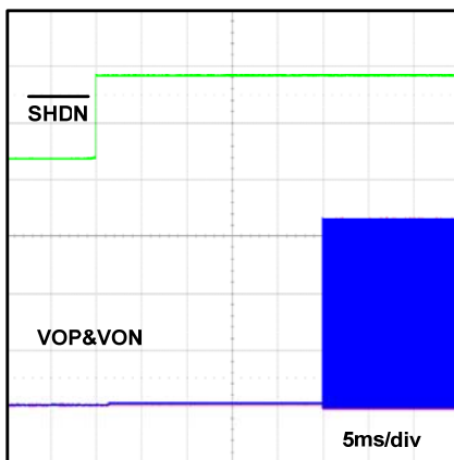
启动时序
