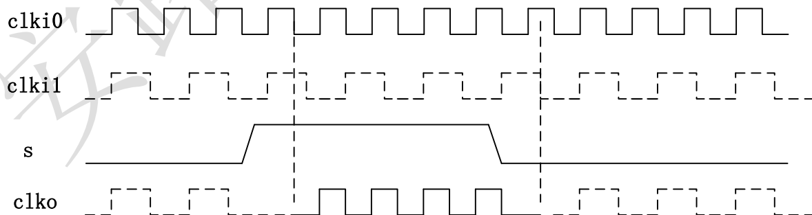
图 2-3-3: CSB 时序图
