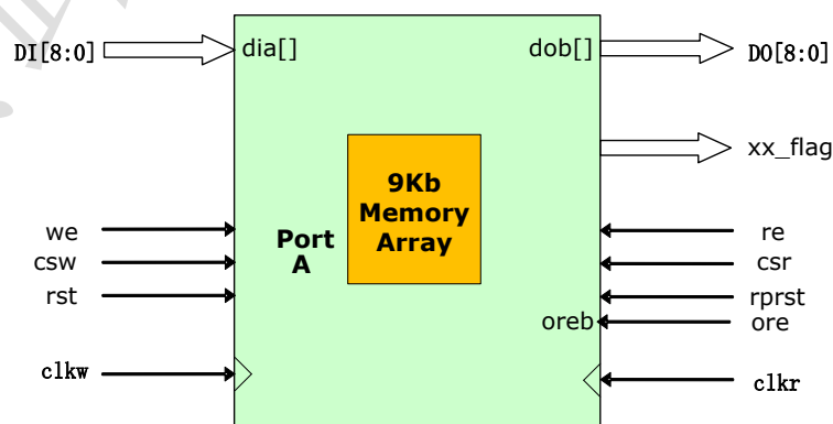
图 2-2-7 \leq 9 位进/ \leq 9 位出 FIFO 模式
