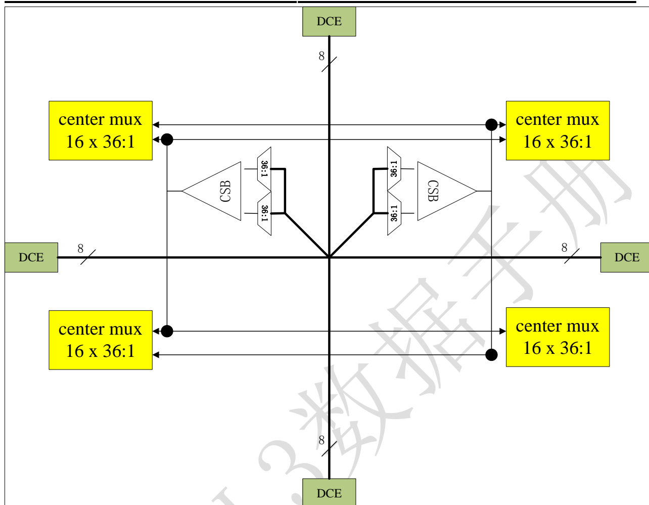
图 2-3-2: CSB 框图
