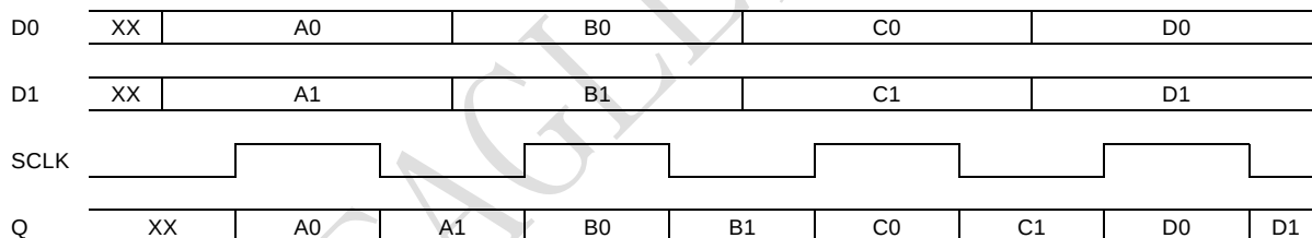
图 2-6-13: Ogddr 输出模式
