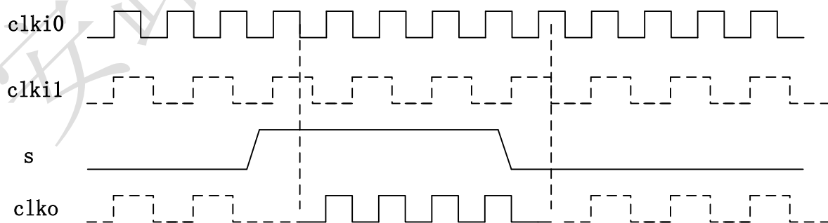
图 2-3-3 : CSB 时序图
