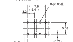
印刷基板加工尺寸 (BOTTOM VIEW) 尺寸公差±0.1mm
