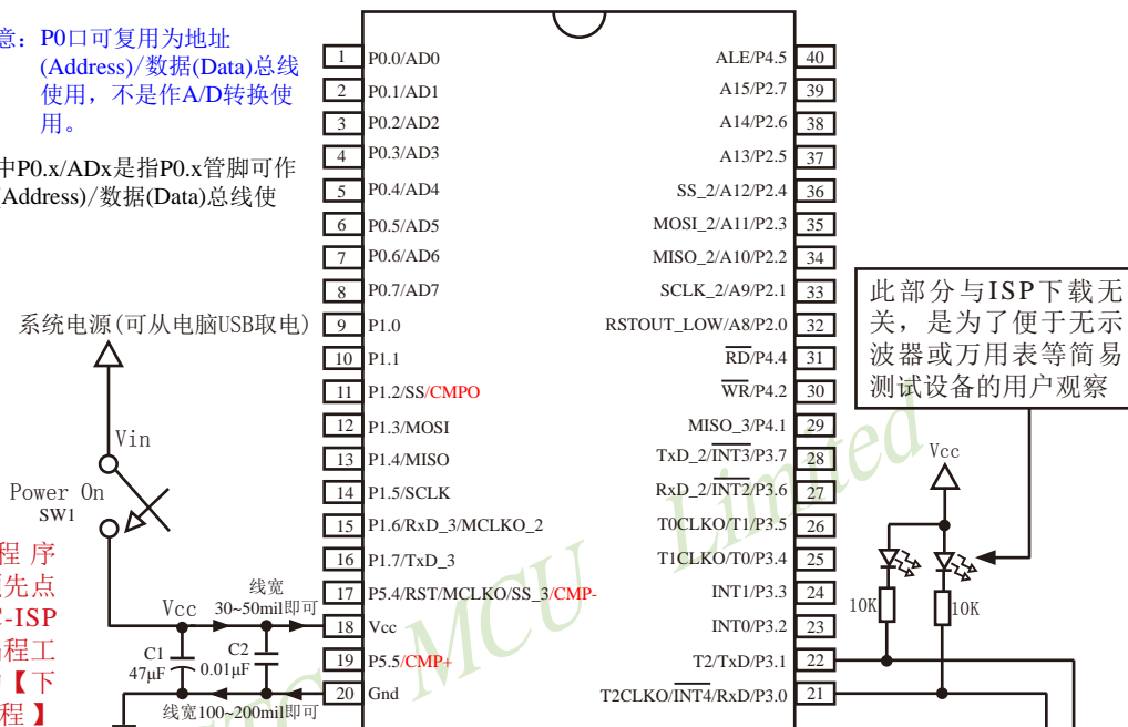
若单片机时钟频率较高, 建议电容C2设置为0.01μF; 若单片机时钟频率较低, 建议电容C2设置为0.1μF
