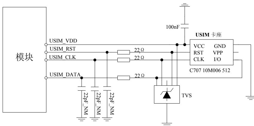
图 19: USIM 接口推荐电路
