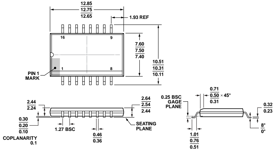
图46. 16引脚标准小型封装, 增加爬电距离[SOIC_IC]
