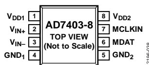
图6. AD7403-8引脚配置
