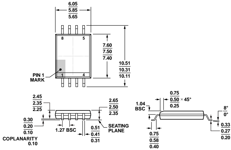
图47. 8引脚标准小型封装, 增加爬电距离[SOIC_IC]
