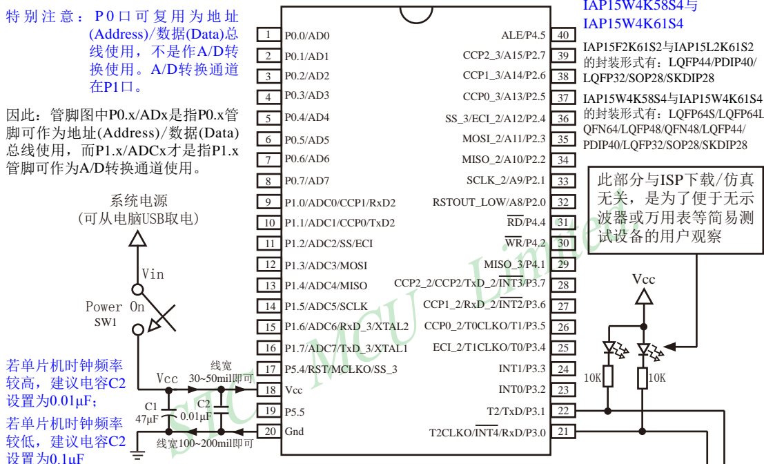
STC 单片机仿真应用线路图
