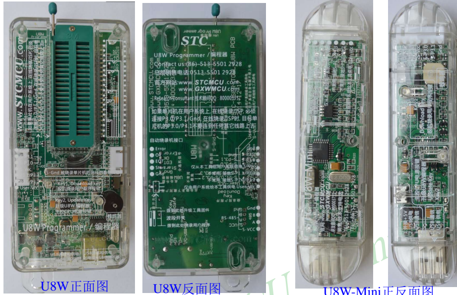
U8W-Mini正反面图
