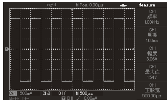
图3-15 屏幕拷贝
