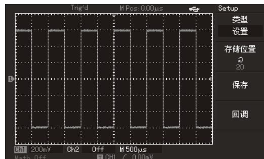
图2-25 设置存储
