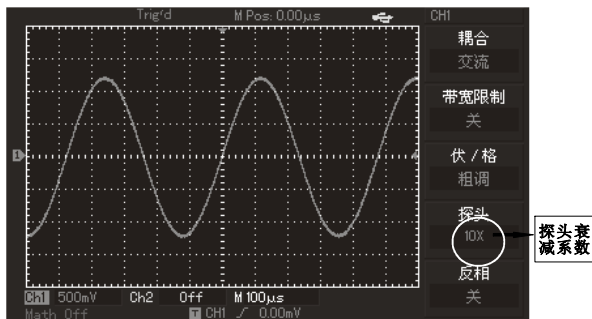
图2-6 通道菜单中的探头衰减系数设定
