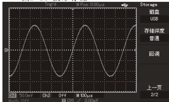
图2-24 用U盘进行波形存储
