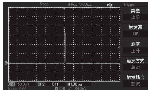
图3-3 单次信号
