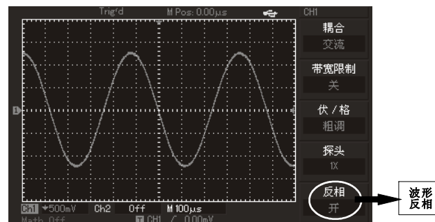
图2-9 垂直通道反相设置（反相）
