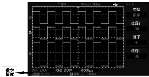
图2-10 数学运算
