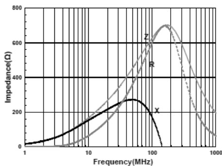
SBH1608S601LSP
