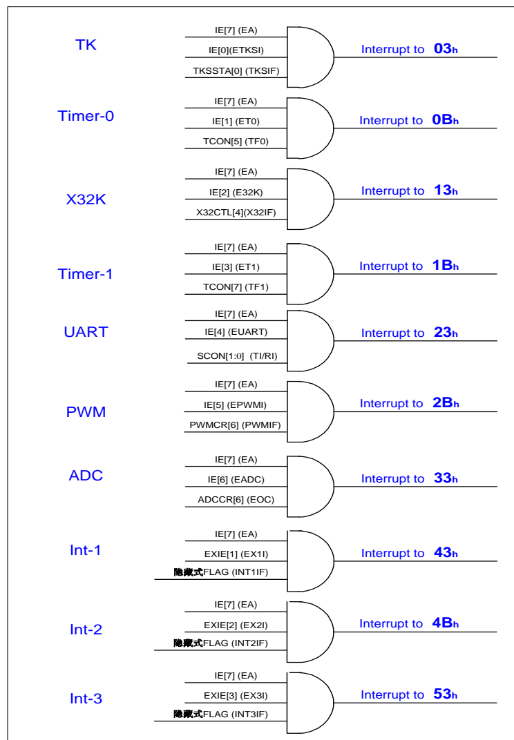
SC91F8311中断结构和向量
