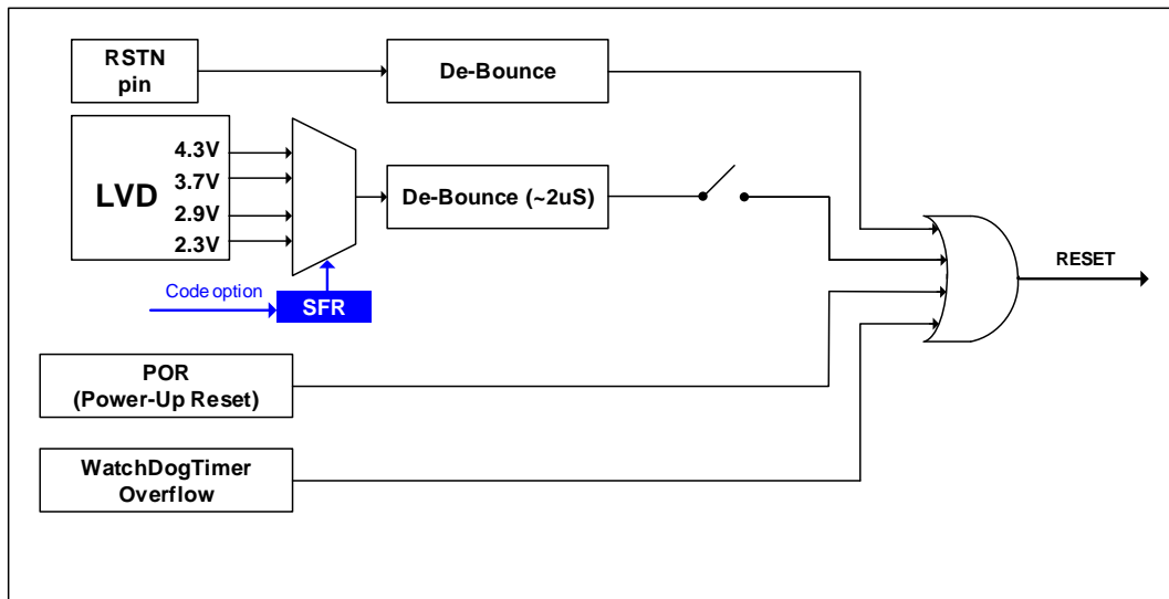
SC92FWXX 复位电路图
