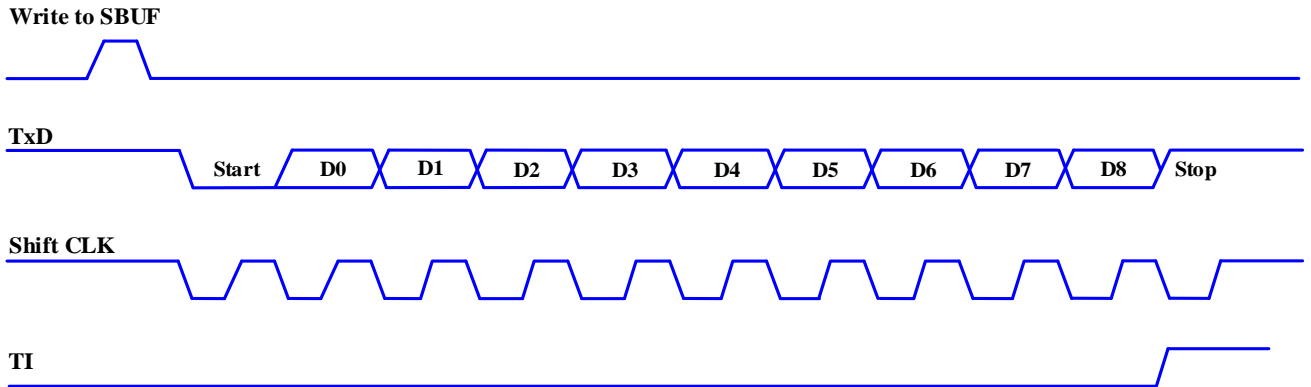
模式3:发送时序图
