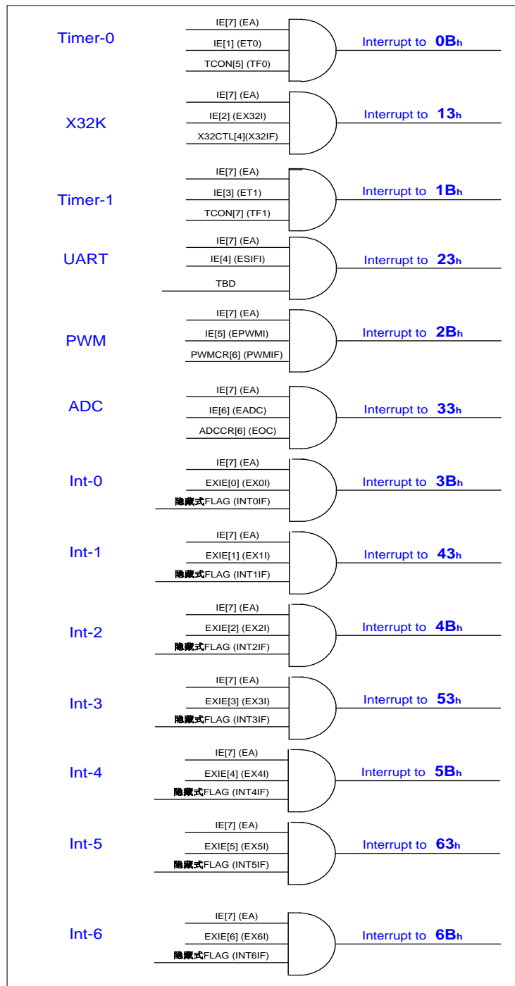
SC91F744 中断结构和向量
