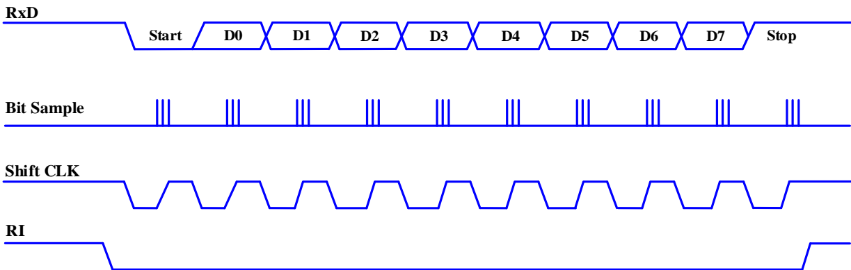
模式1:接收时序图
