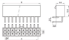
双排穿针座 WAFER(5569)
