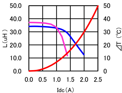
CDRH70D45BT150NP-101MC
