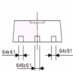
SOT89-3
