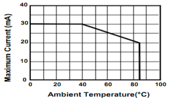
8).Thermal Design
