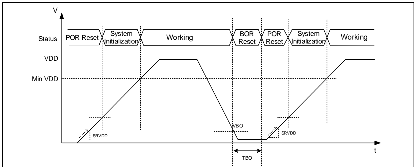
Figure 16-2 上电和掉电示意图
