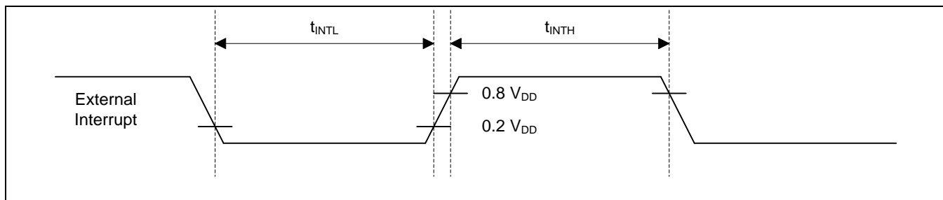
Figure 16-3 外部中断输入时序
