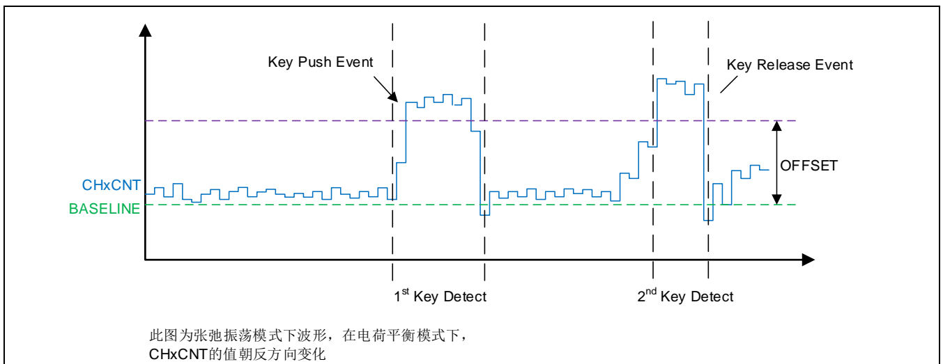
Figure 15-4 按键触发示意图
