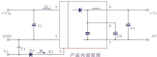
单路输出
