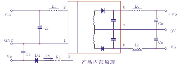
正负双路
