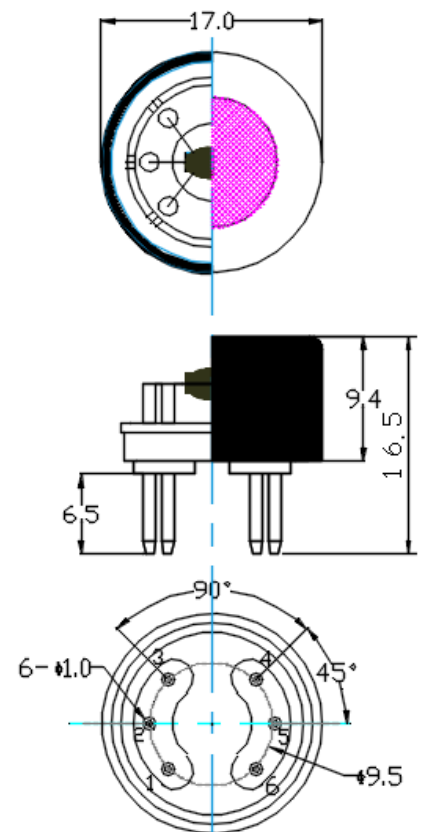
图中未标注尺寸单位: mm 未标注尺寸公差: ±0.1mm
