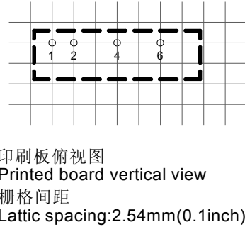
建议印刷板图
