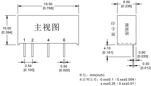
封装尺寸图
